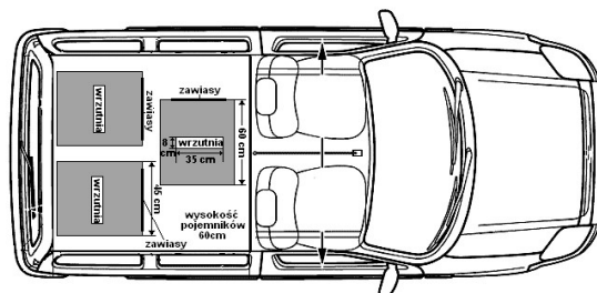
Bankowóz typu C wyposażony w 3 jednakowe pojemniki klasy D
